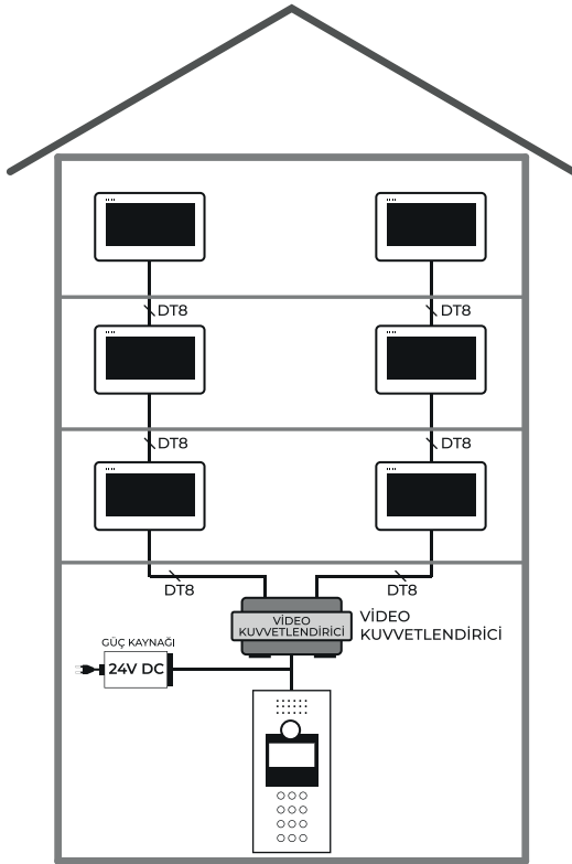
MULTIBUS DAİREDEN DAİREYE GEÇİŞLİ UYGULAMADA KABLOLAMA
