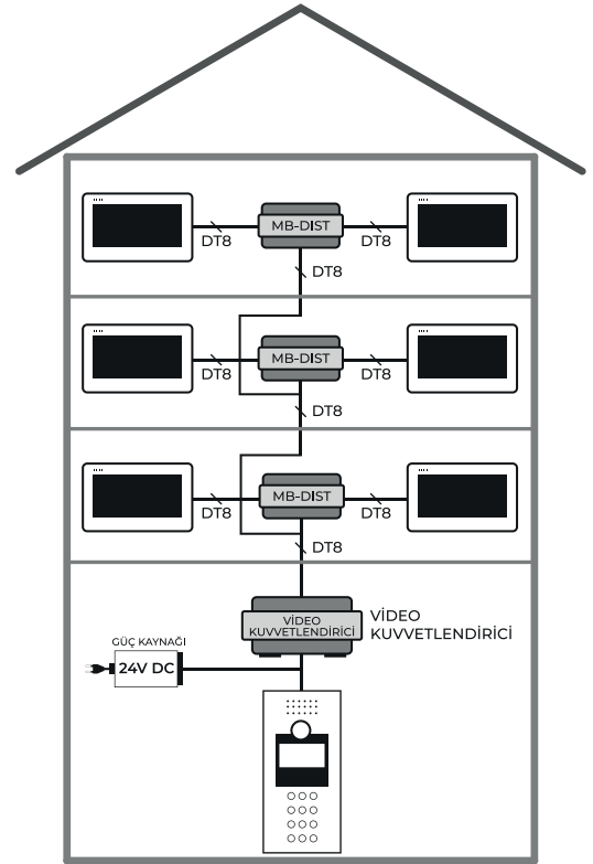
MULTIBUS BUAT TİPİ UYGULAMADA KABLOLAMA
